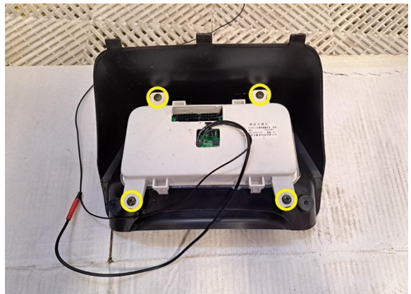
Irrota mittariston kehyksessä kiinni pitävät kiinnitysruuvit. (ristipäämeisseli ph2).
